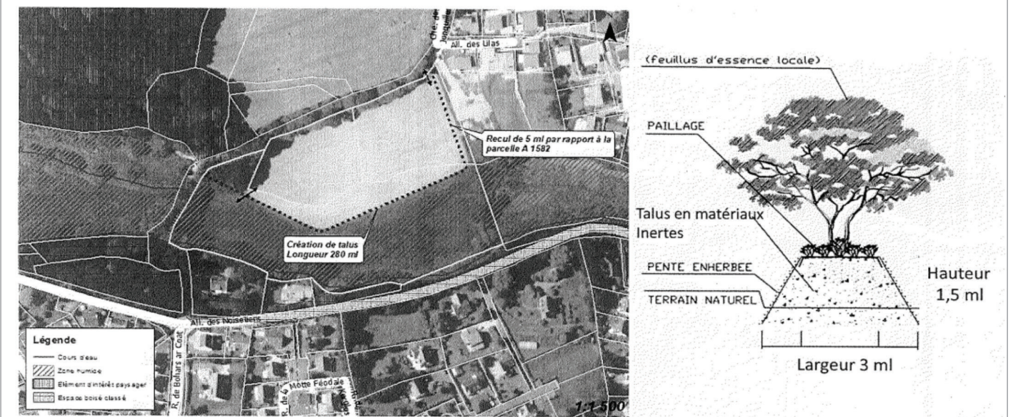
Implantation et coupe du talus à créer
